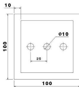
Front view Scale: 1:1
